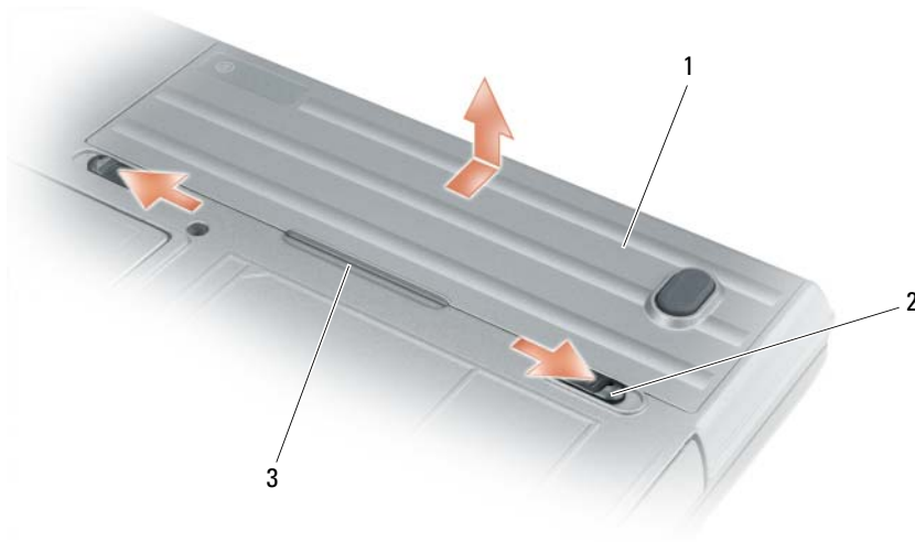
1 batterij 2 ontgrendelingsschuifjes van batterijcompartiment (2) 3 batterijlipje
